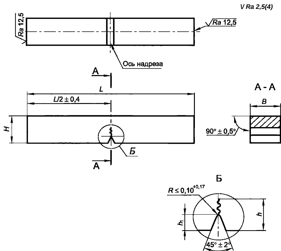
Рисунок 3 — Образец с концентратором вида Т (усталостная трещина)
